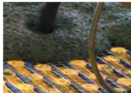
Massetto di calcestruzzo su pavimento radiante
