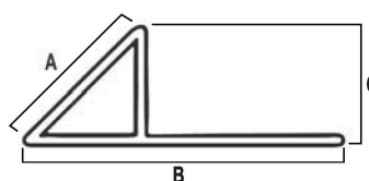
SMUSSO PER PILASTRI ALETTATO - barre da 2 mt
