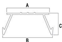
GOCCIOLATOIO PER BALCONI - barre da 2 mt
